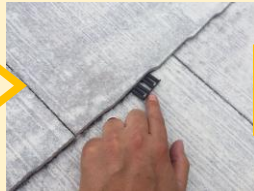
下塗り後 タスペーサー施工
